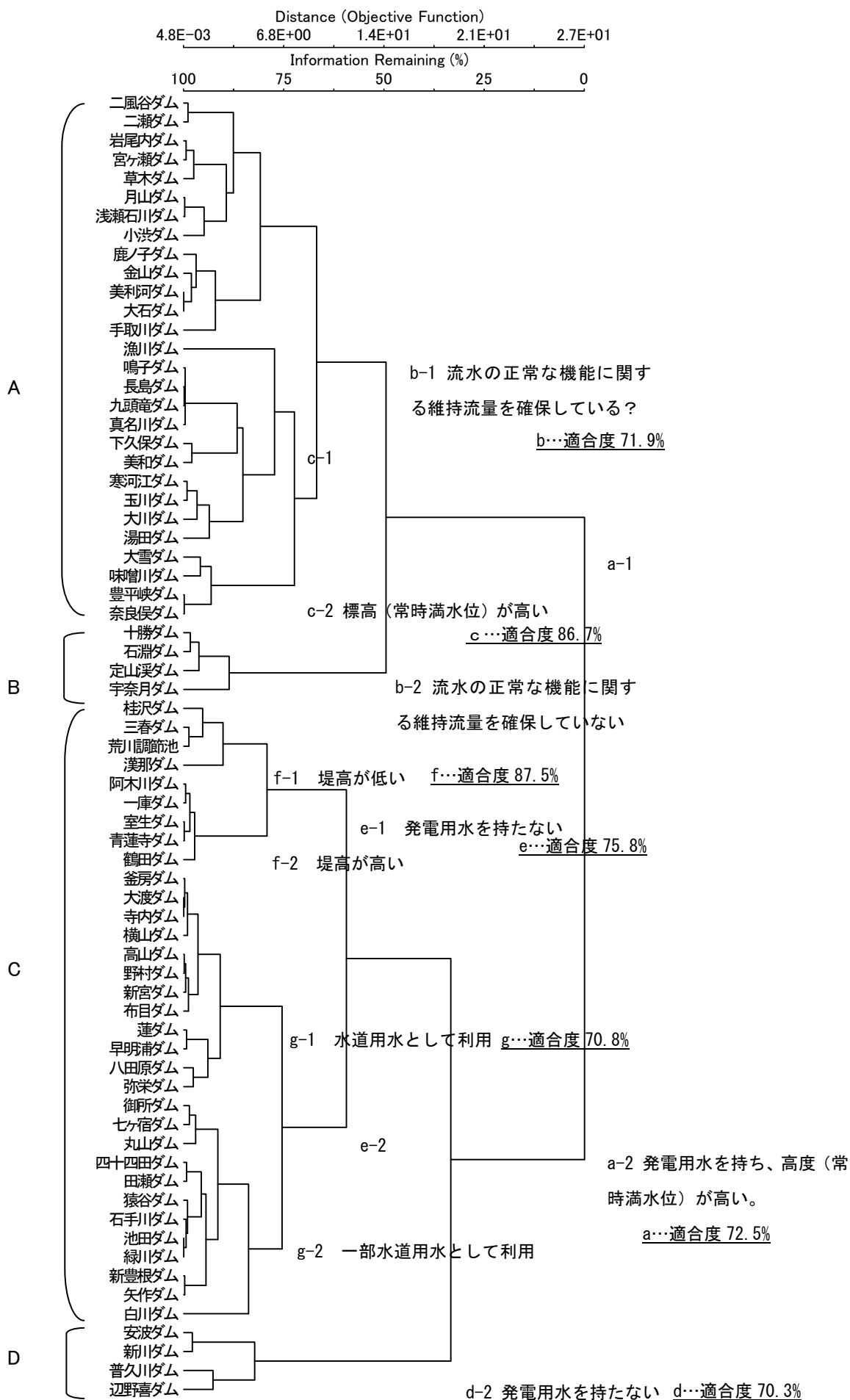
図.ダム湖に出現する魚類の生息環境評価を用いた主成分得点のクラスター分析と判別分析
